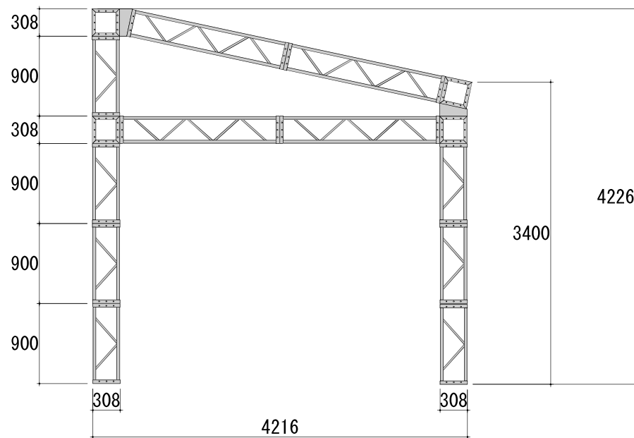
■側面図
