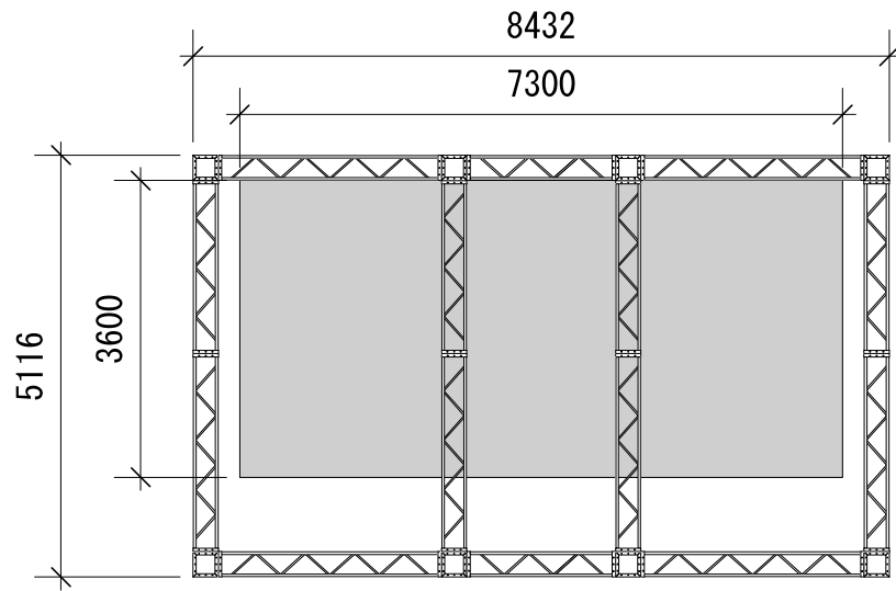
■平面
